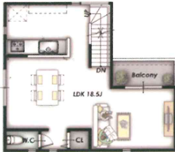
2Fplan
